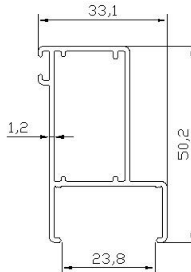
08 ALP 941 - 0.536 Kg/m
