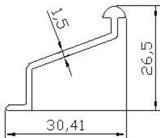
08 ALP 940 - 0.215 Kg/m
