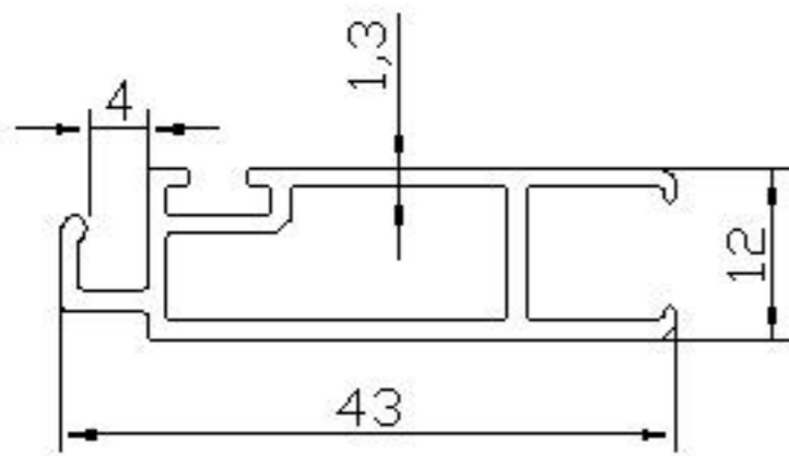
08 ALP 946 - 0.398 Kg/m
