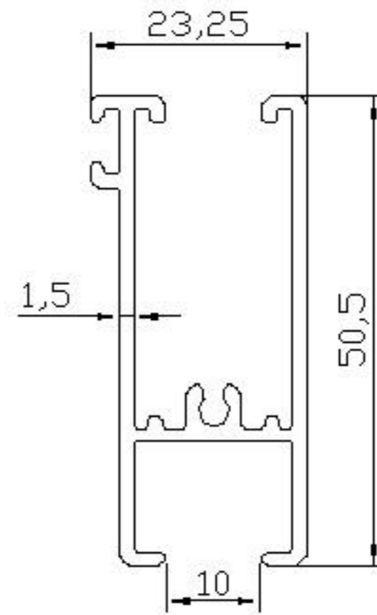
08 ALP 945 - 0.619 Kg/m
