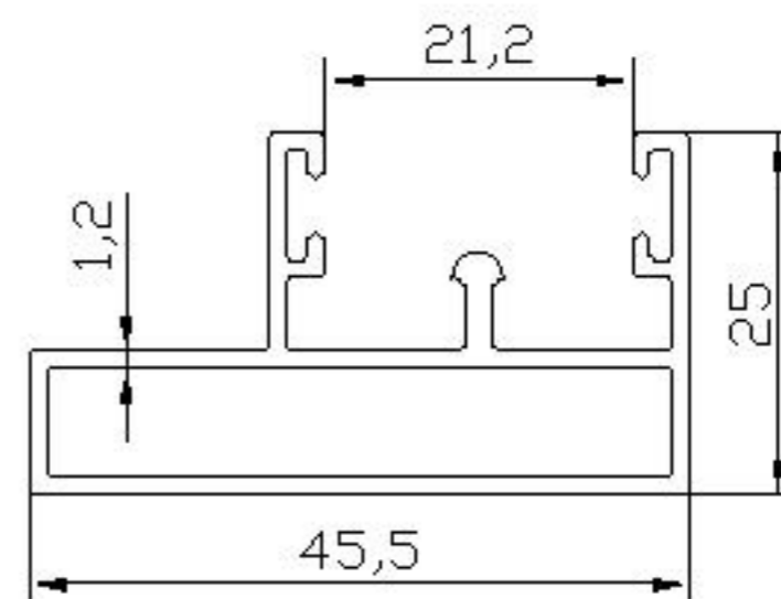
08 ALP 883 - 0.546 Kg/m
