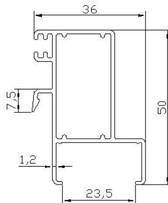
08 ALP 942 - 0.603 Kg/m
