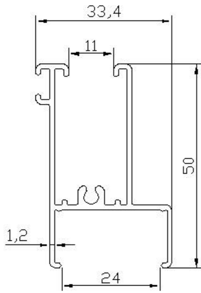
08 ALP 944 - 0.542 Kg/m
