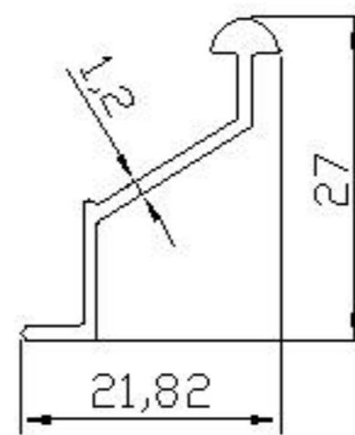
08 ALP 939 - 0.159 Kg/m
