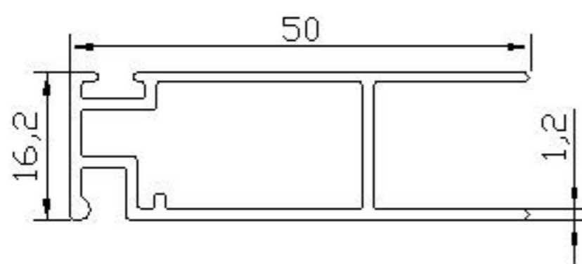
08 ALP 884 - 0.463 Kg/m
