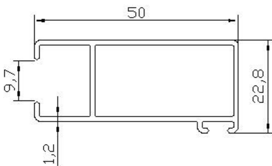
08 ALP 948 - 0.491 Kg/m
