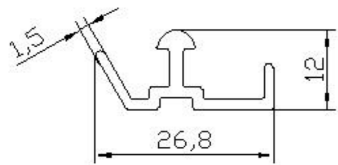
08 ALP 938 - 0.231 Kg/m
