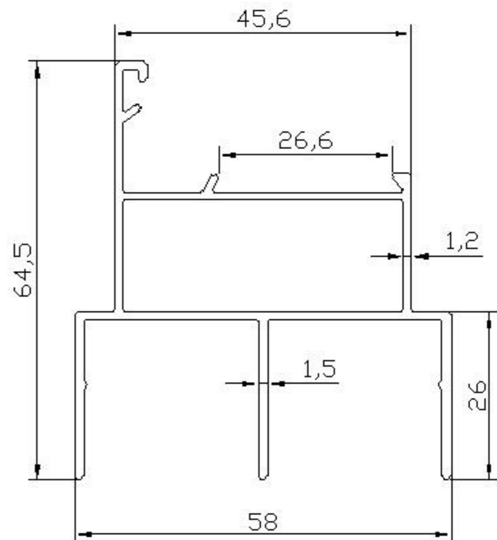
08 ALP 947 - 0.875 Kg/m
