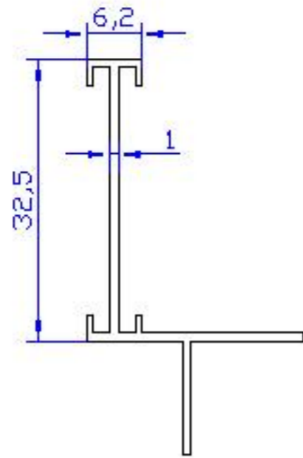
07 ALP 365 - 0.215 Kg/m
