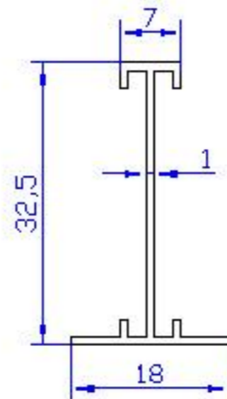
07 ALP 369 - 0.172 Kg/m
