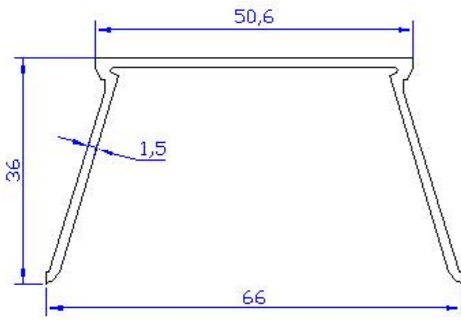
07 ALP 240 - 0.503 Kg/m
