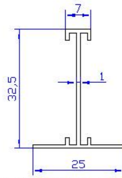
07 ALP 237 - 0.191 Kg/m
