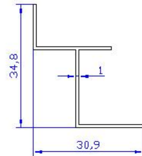
07 ALP 370 - 0.180 Kg/m
