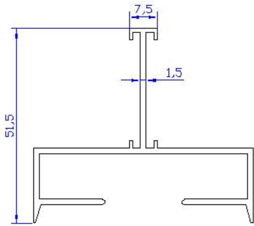
07 ALP 236 - 0.685 Kg/m
