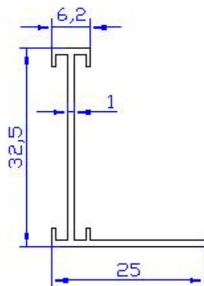
07 ALP 367 - 0.180 Kg/m
