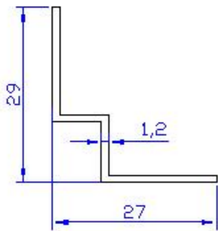
07 ALP 366 - 0.178 Kg/m
