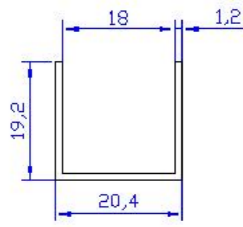
07 ALP 235 - 0.183 Kg/m
