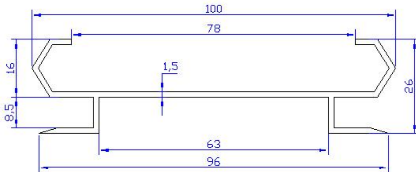
07 ALP 239 - 0.730 Kg/m
