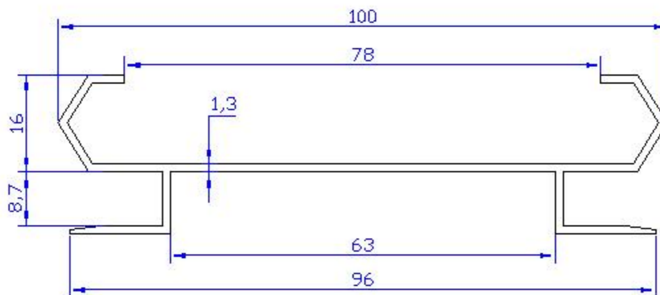
07 ALP 242 - 0.643 Kg/m
