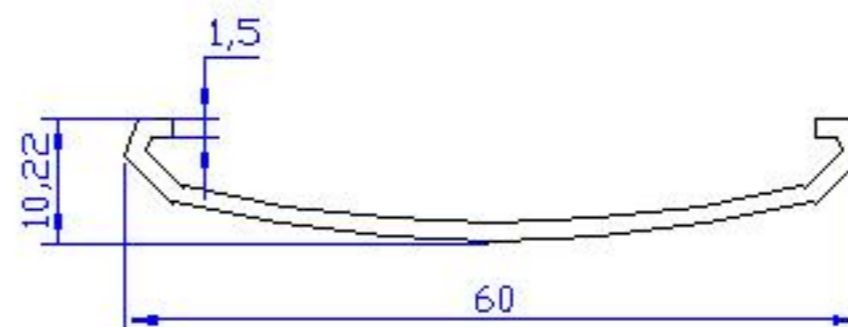
07 ALP 243 - 0.288 Kg/m
