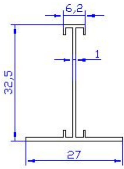
07 ALP 234 - 0.186 Kg/m
