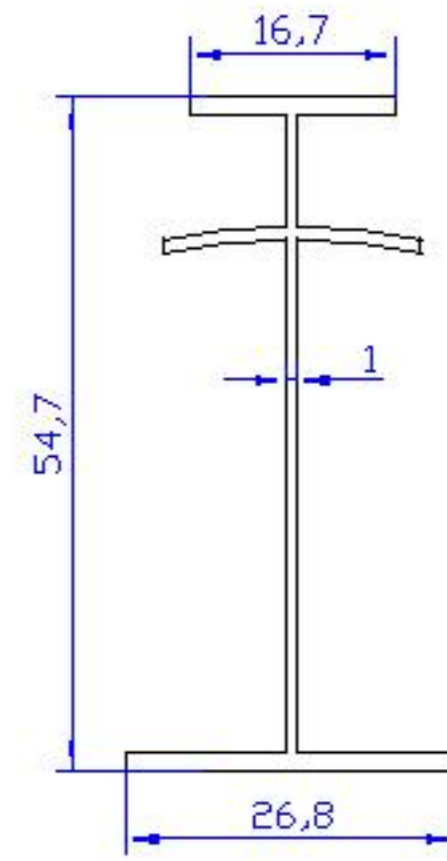
07 ALP 241 - 0.370 Kg/m
