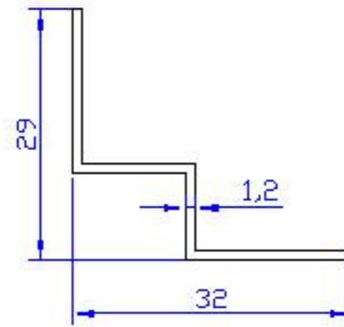
07 ALP 368 - 0.194 Kg/m
