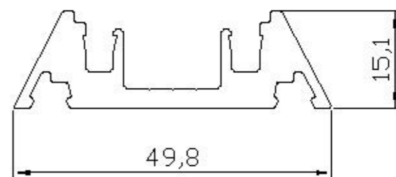
07 ALP 229 - 0.812 Kg/m
