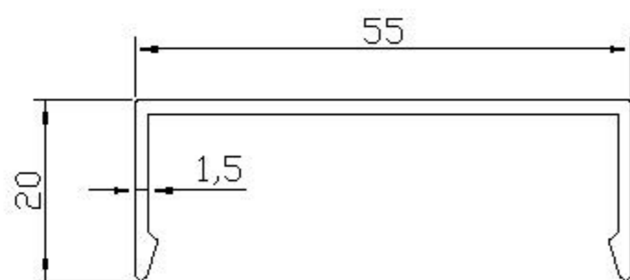
07 ALP 223 - 0.385 Kg/m
