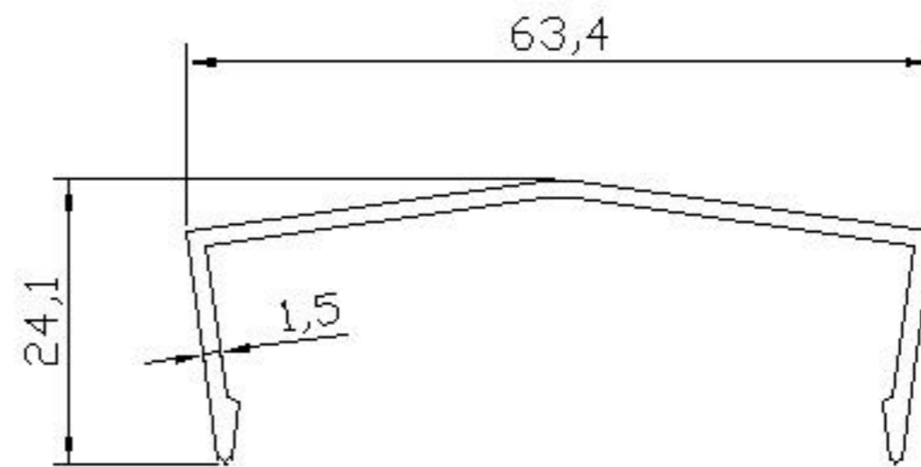
07 ALP 225 - 0.415 Kg/m
