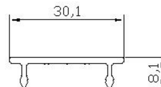
07 ALP 228 - 0.173 Kg/m
