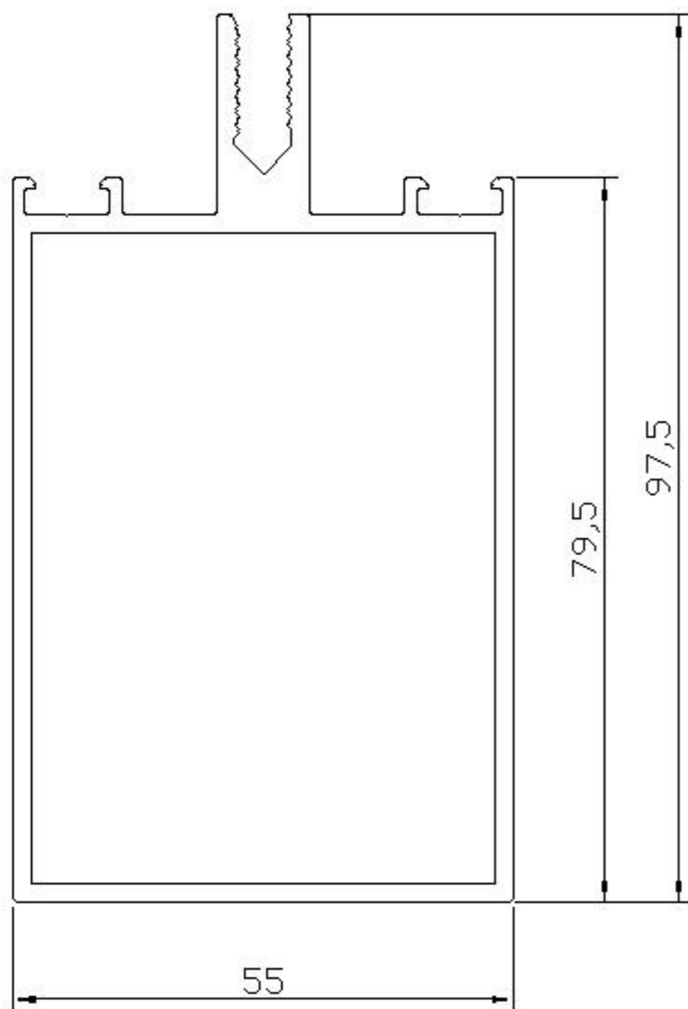
07 ALP 222 - 1.780 Kg/m
