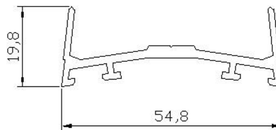
07 ALP 226 - 0.549 Kg/m
