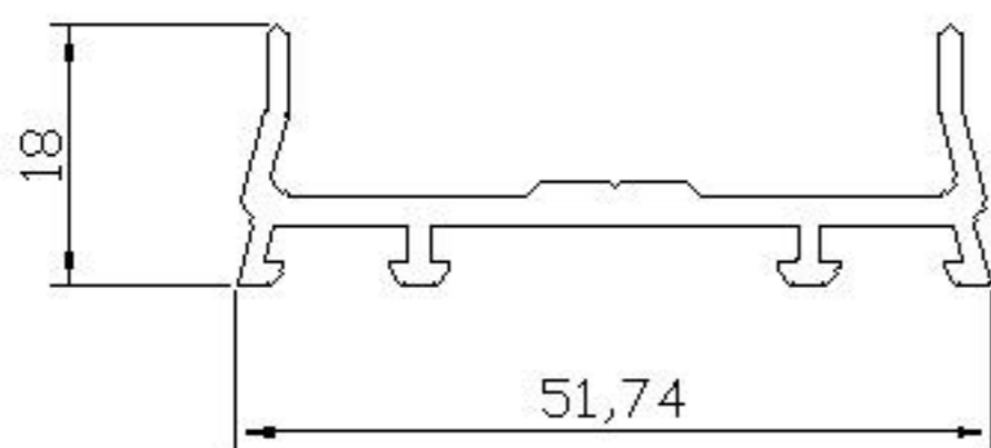
07 ALP 224 - 0.501 Kg/m
