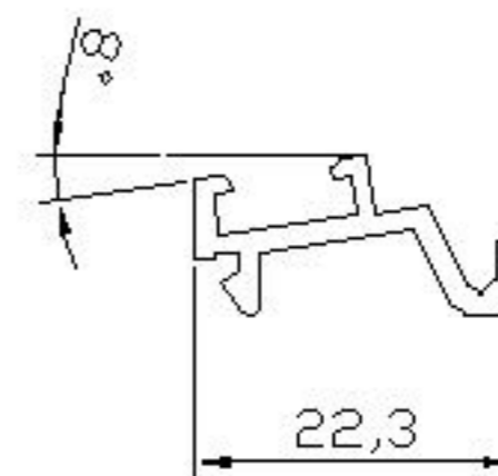
07 ALP 227 - 0.176 Kg/m
