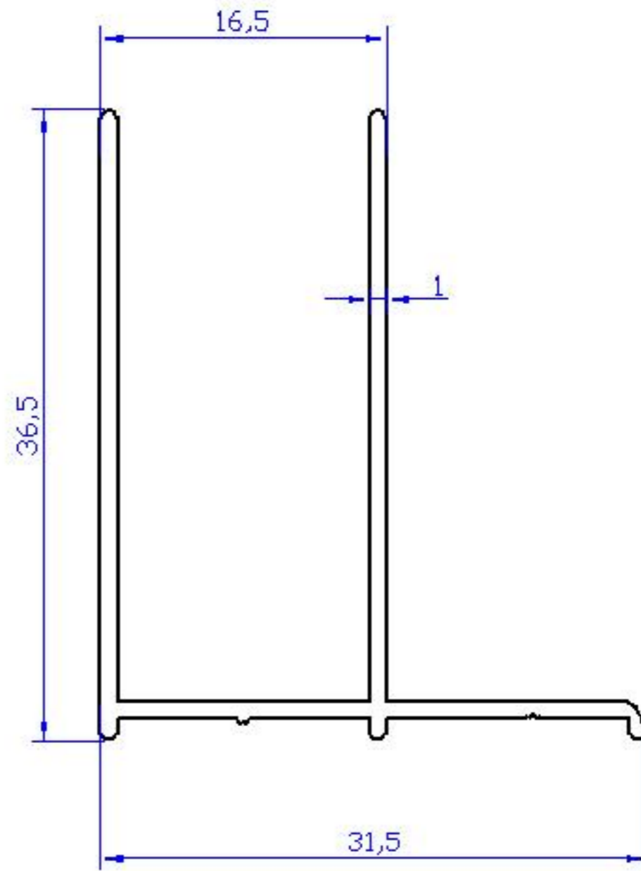
07 ALP 111 - 0.279 Kg/m
