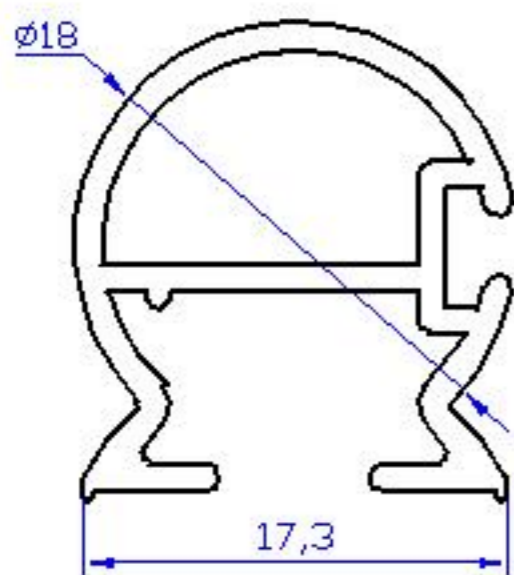
07 ALP 102 - 0.240 Kg/m
