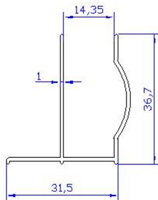
07 ALP 100 - 0.284 Kg/m
