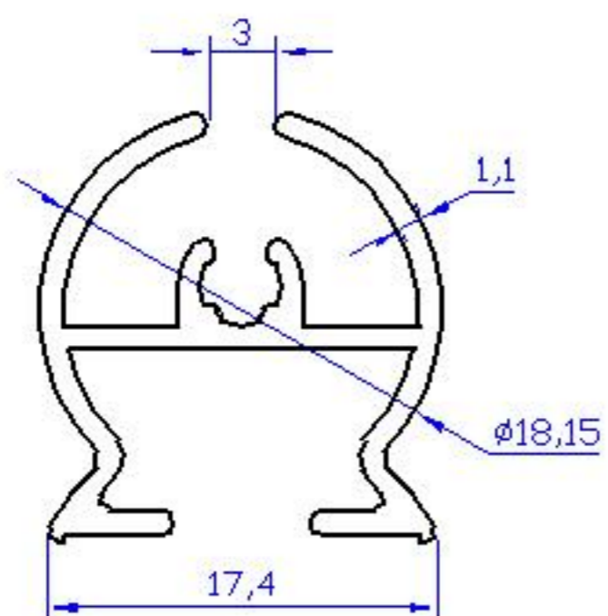
07 ALP 104 - 0.235 Kg/m
