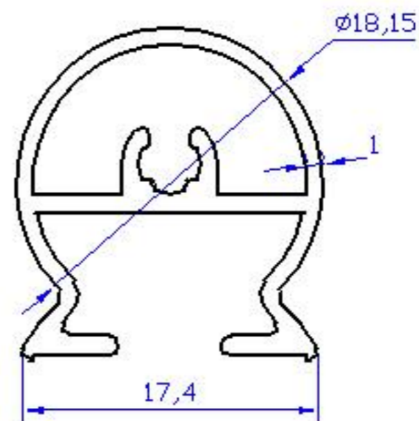
07 ALP 103 - 0.235 Kg/m
