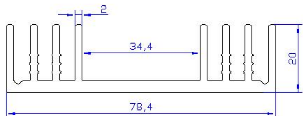
07 ALP 462 - 1.460 Kg/m
