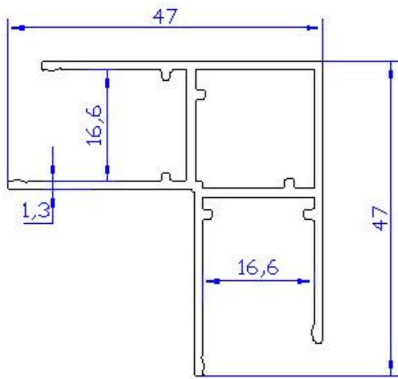
07 ALP 511 - 0.649 Kg/m
