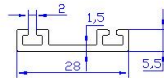
08 ALP 770 - 0.203 Kg/m
