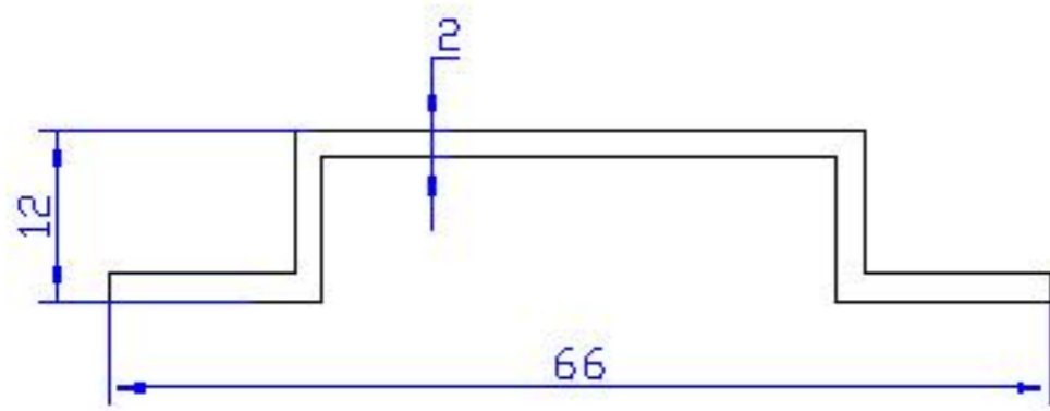
07 ALP 551 - 0.466 Kg/m
