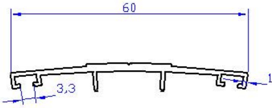
07 ALP 549 - 0.315 Kg/m
