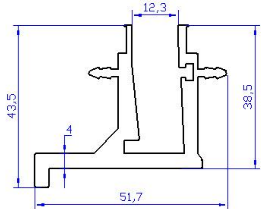
08 ALP 895 - 1.355 Kg/m
