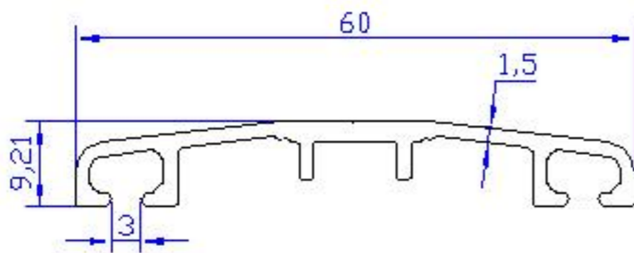
08 ALP 914 - 0.439 Kg/m
