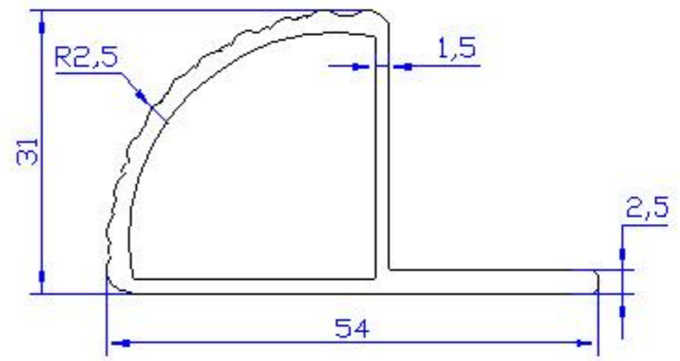
08 ALP 734 - 0.659 Kg/m
