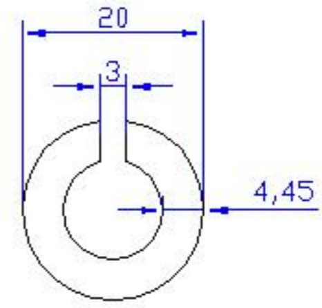
08 ALP 725 - 0.553 Kg/m
