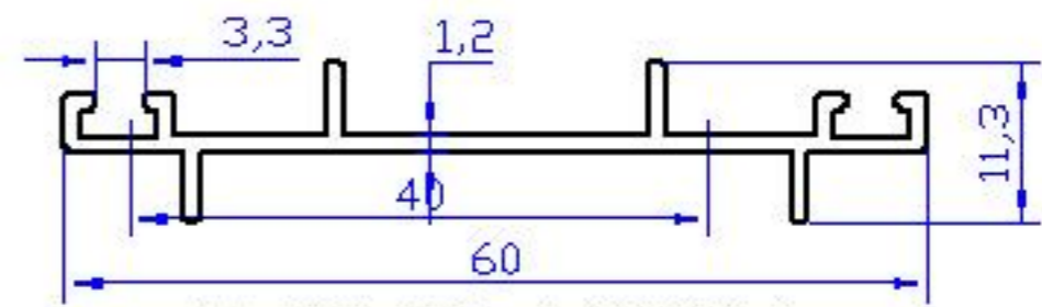
07 ALP 548 - 0.304 Kg/m
