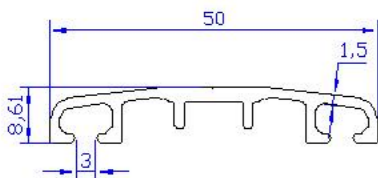
08 ALP 839 - 0.398 Kg/m
