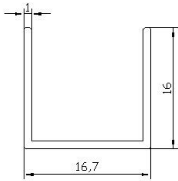
08 ALP 835 - 0.126 Kg/m
