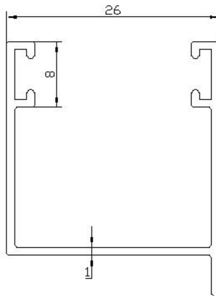
08 ALP 837 - 0.259 Kg/m
