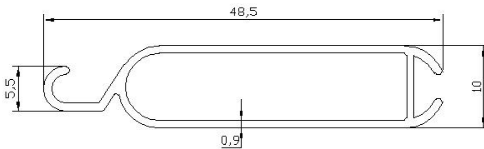
08 ALP 836 - 0.272 Kg/m
